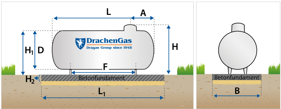
Abmessungen Betonfundament (Mindestmaße)
