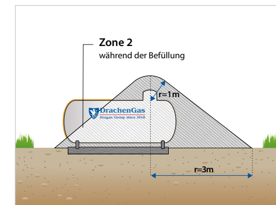
Oberirdische Aufstellung
