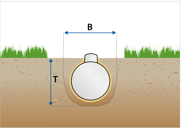
Maßtabelle Einlagerungsgrube
