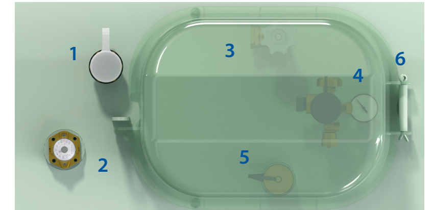
Beispiel: oberirdischer Behälter
