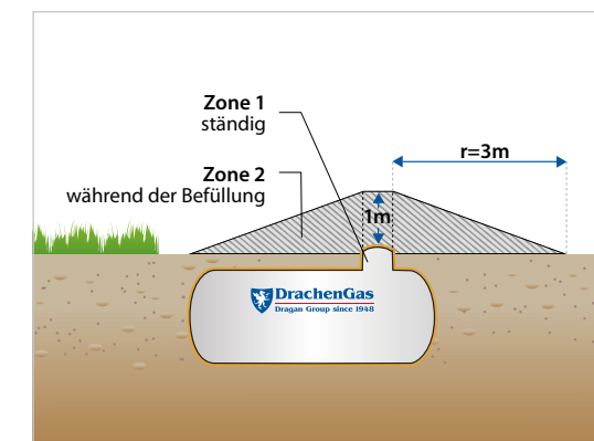
Unterirdische Einlagerung
